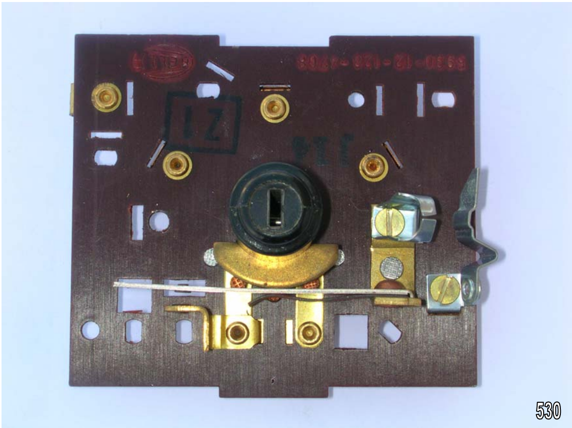
Detalle de la placa eléctrica marca Hella, por ambas caras
